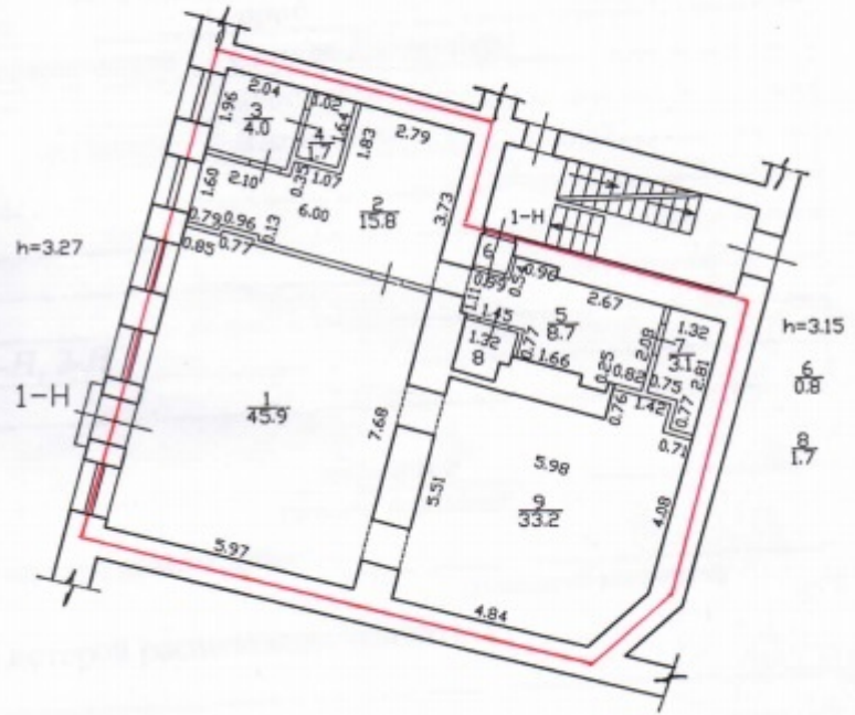
План 1 этажа
