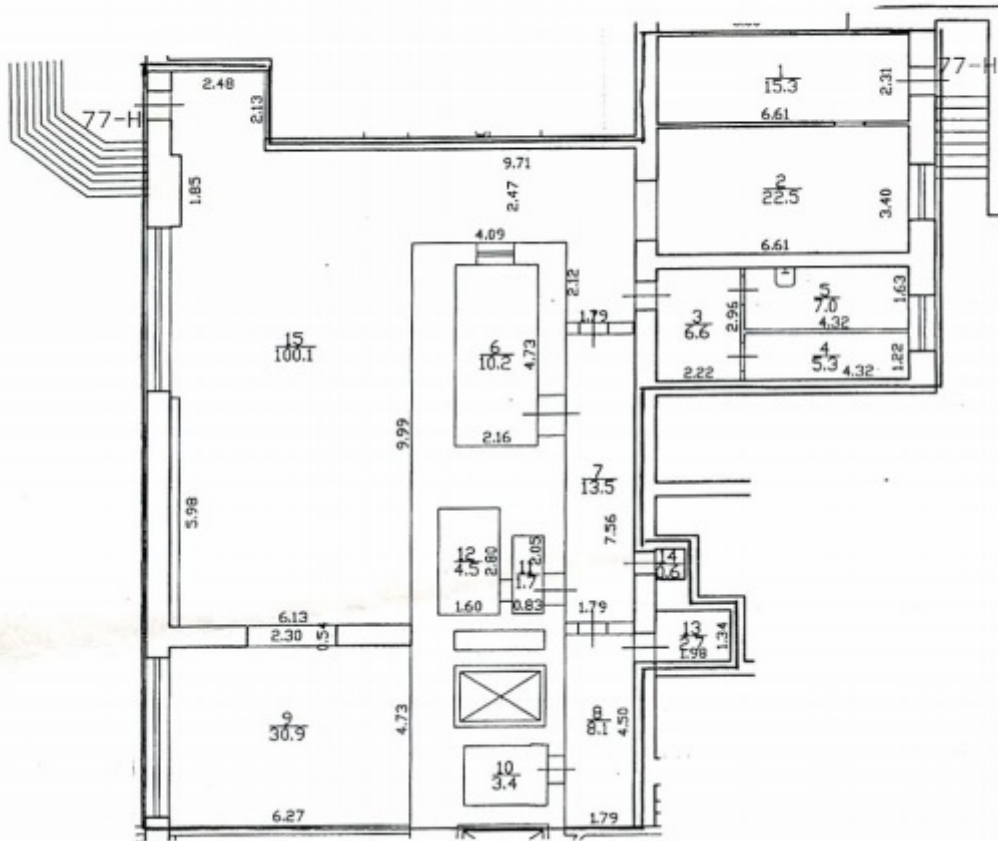
План 1 этажа
