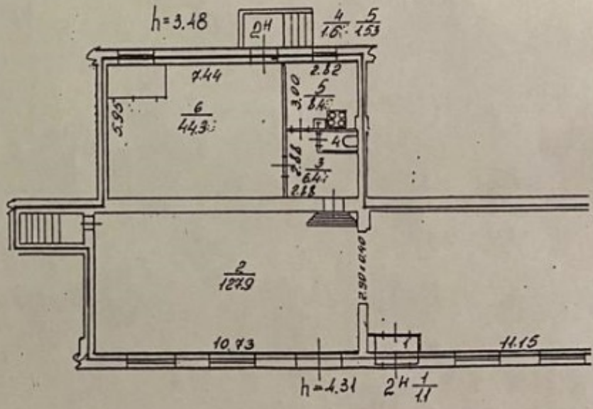
План 1 этажа
