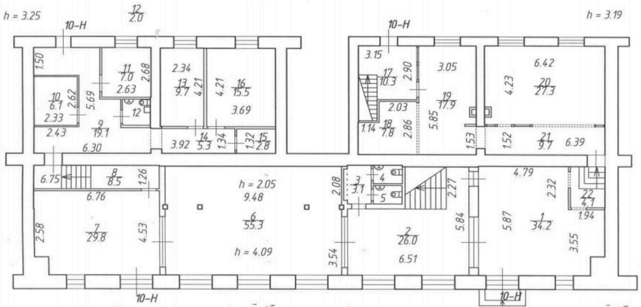
План 1 этажа
