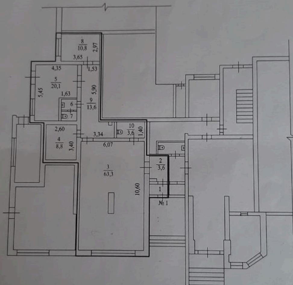
План 1 этажа
