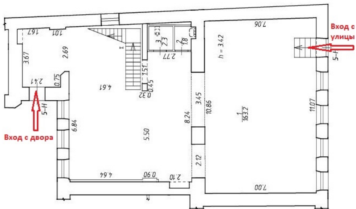
ПЛАН ЧАСТИ 1 ЭТАЖА
