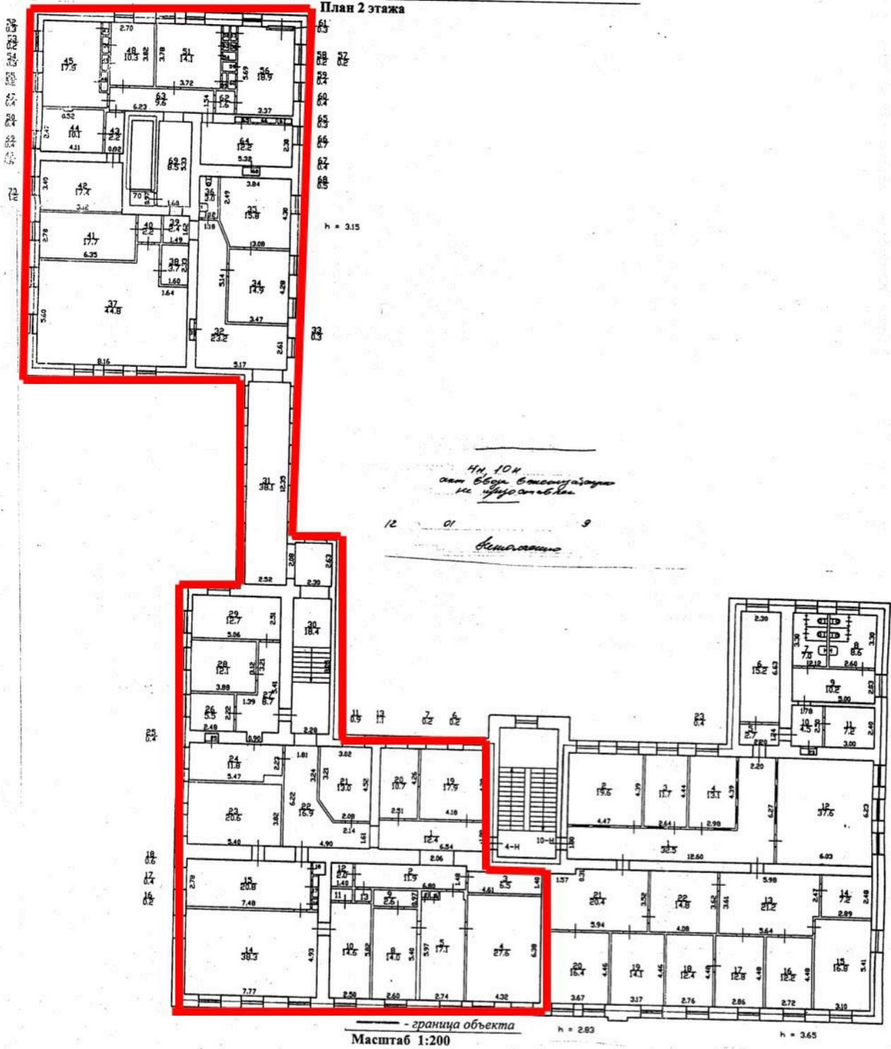
План 2 этажа
